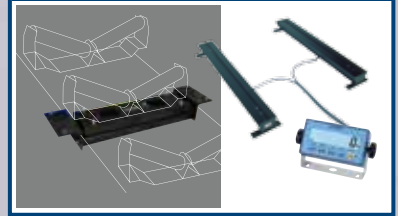
PESATURA PER NASTRI TRASPORTATORI
